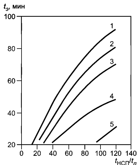
Рисунок Р.3 — Зависимость эквивалентной продолжительности пожара t_{э} от продолжительности пожара для железобетонных и огнезащищенных металлических конструкций перекрытия в условиях локальных пожаров t_{л} (или продолжительности НСП t_{нсп} ) при горении твердых и трудногорючих материалов
